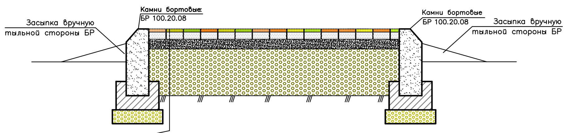
Узел бортового камня БР 100.20.8
